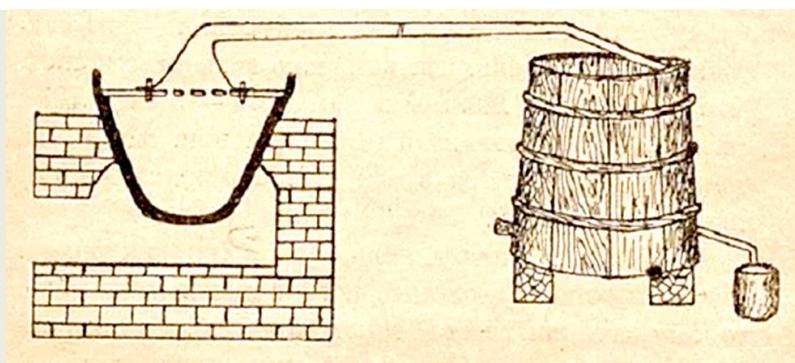
Аппарат для сухой перегонки древесины /32/.
